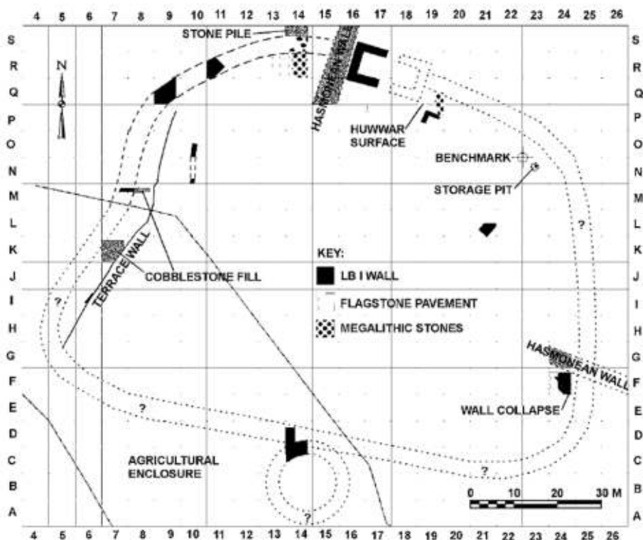
Рис. 3. Схема крепости периода поздней бронзы I в Хирбет эль-Макатире 22
